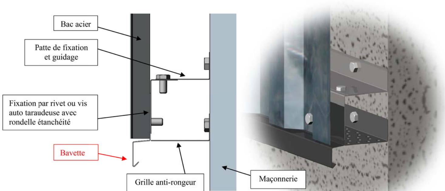
Montage bavette avec grille anti-rongeur
