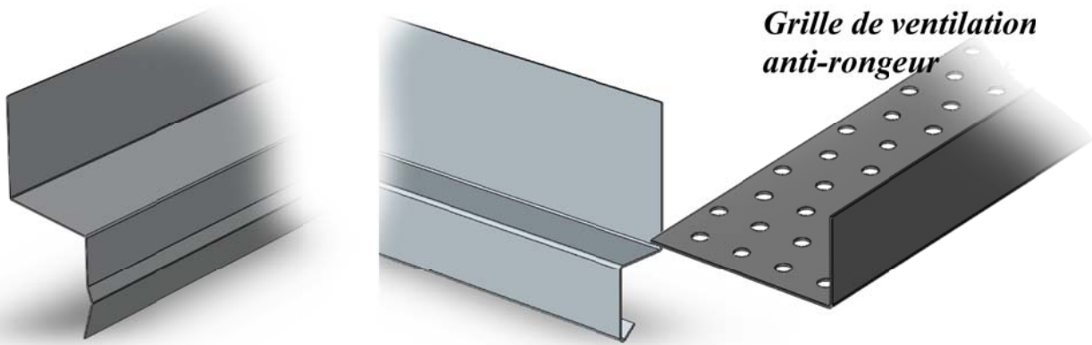
Montage bavette avec grille anti-rongeur
