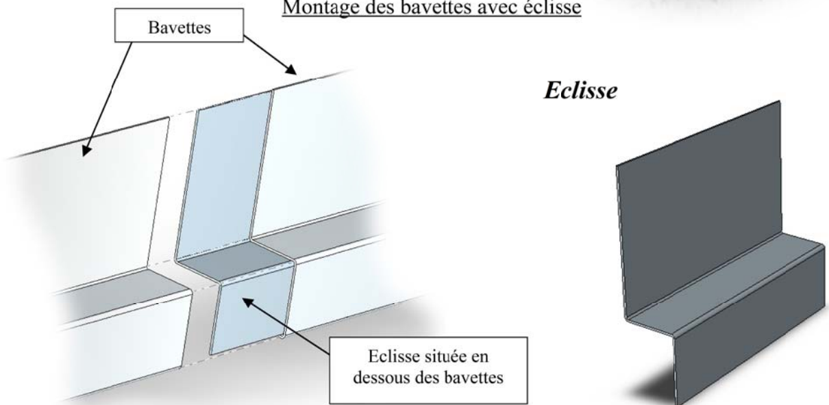
Montage des bavettes avec éclisse
