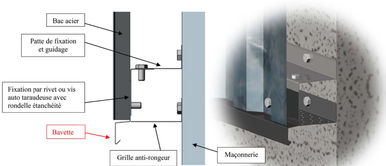
Montage des bavettes avec éclisse
