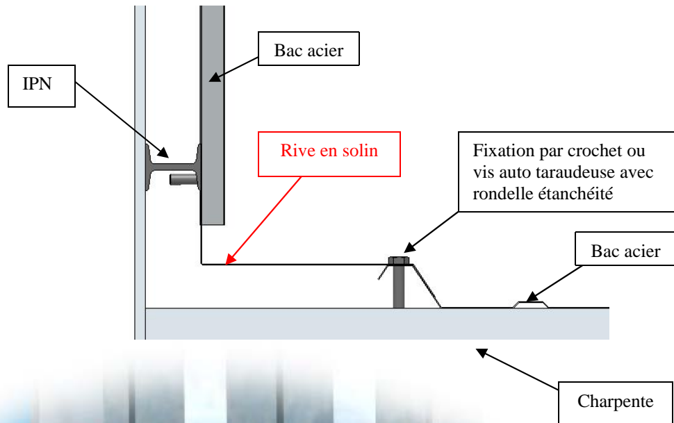
Montage rive en solin
