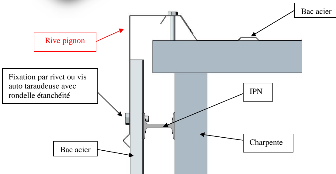
Montage rive pignon
